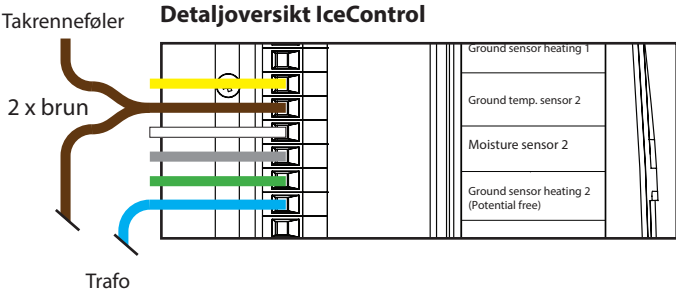
Detaljoversikt tilkobling
