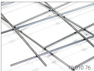
TF STÅLNETT 0,77 x 1,17 meter Maskevidde er 6,7 cm. TF stålnett er spesielt godt egnet i kombinasjon med Hey'di sparkelmasser både for å avstive og forsterke gulvkonstruksjonen med bjelkeavstand c/c 60.
